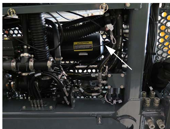
Vanne de vidange du réservoir (de purge de l'air) - si la machine en est équipée (situé sous la plate-forme d'entretien, dans la partie centrale de la machine)
