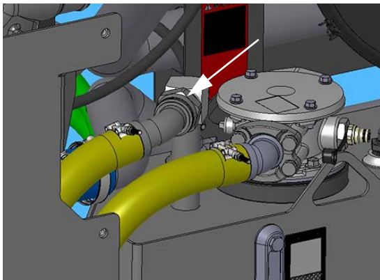
Tuyau de vidange du carter (situé près du haut du réservoir d'huile hydraulique) - Vue typique
