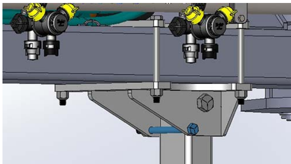
Boulon de maintien remis en place - Vue typique
