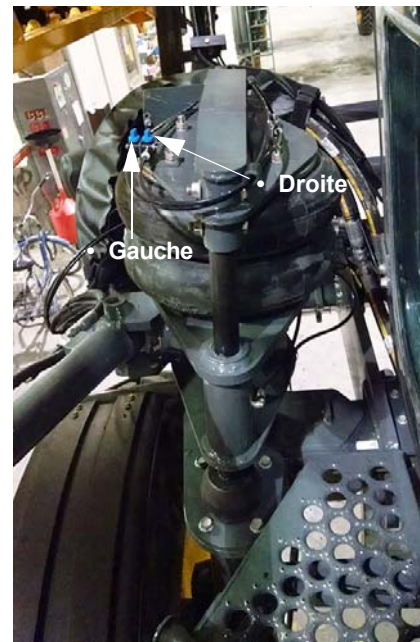
Vannes de la suspension pneumatique (situées sur le coussin d'air gauche avant)
