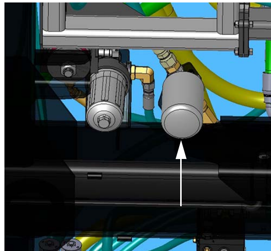
Filtre de retour au carter 2 (situé sur le côté gauche de la machine, à l'avant du châssis du moteur) - Vue typique
