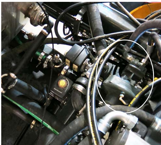
Pompe à solution (située dans la partie centrale de la machine) - Vue typique
