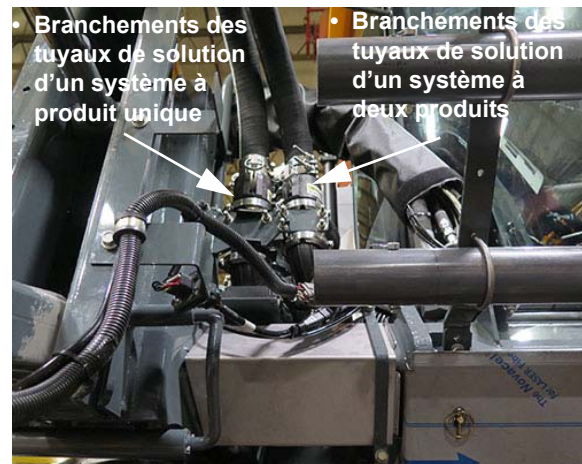
Branchements des tuyaux de solution - Produit unique/Deux produits (situé à l'avant droit de la machine) - Vue typique
