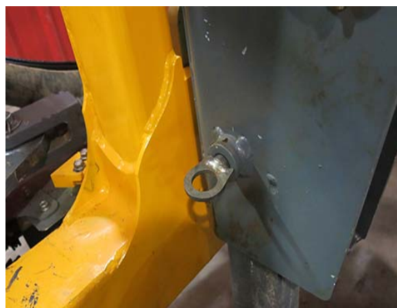
Goupille de verrouillage retirée - Vue typique
