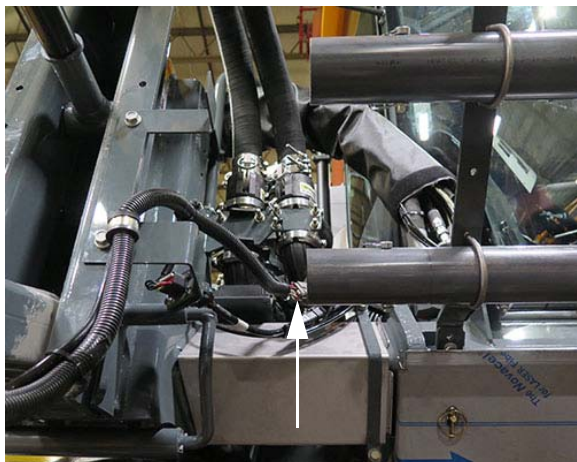
Branchements électriques d'un système à deux produits - si la machine en est équipée (situé à l'avant droit de la machine) - Vue typique
