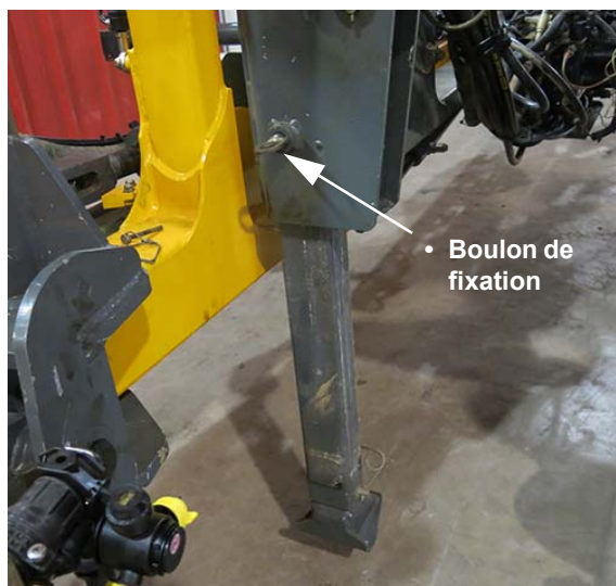
• Boulon de fixation Chandelle de support de la rampe (illustrée en position étirée) - Vue typique
