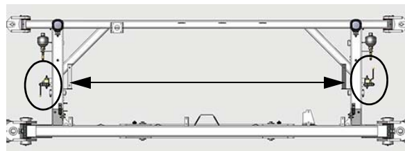
Vannes manuelles NORAC (2) Rampe hybride de 36 mètres (situées à côté du vérin au niveau de chaque côté de la traverse) - Vue typique
