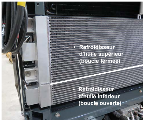
Refroidisseur d'huile (situé sur la partie avant du moteur - retirer la calandre pour y accéder) - Vue typique
