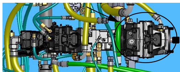
Pompe hydrostatique (pompe d'entraînement) - Vue typique (Vue depuis le dessus de la machine)
