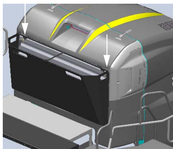
Brides à ressort de la prise d'air du moteur (situées en haut à gauche et à droite de la prise d'air intérieure) - Vue typique
