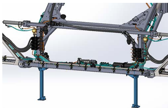
Chandelles de support de la rampe - Vue typique
