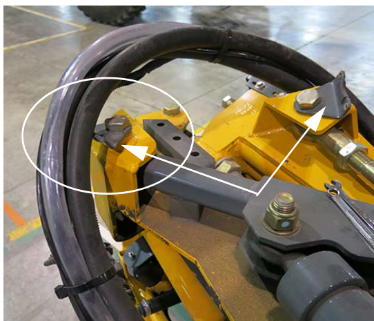
Supports d'acheminement des tuyaux flexibles (2) (situés près de l'extrémité des extensions extérieures de la rampe) - Vue typique
