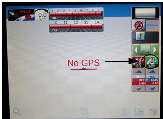
Interrupteur de pompe à solution - Secondaire (situé sur la console du système de pulvérisation) - Vue typique
