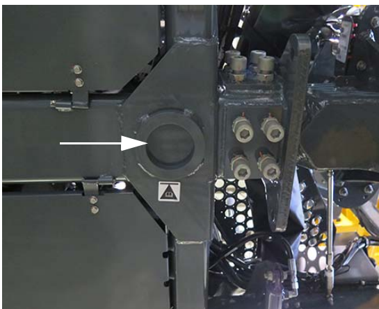
Anneau de rétention du point de levage (situé sur le châssis, près de chaque jambe) - Vue typique
