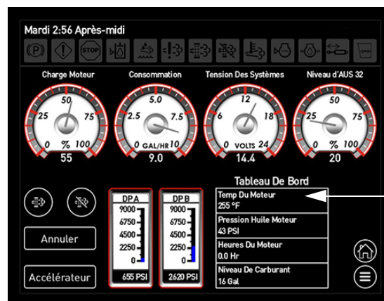
Température du liquide de refroidissement du moteur (située sur l'écran Diagnostique du moteur)
