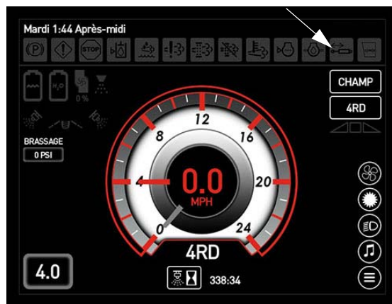
Indicateur de pression dans la rampe (situé sur la page d'accueil de l'afficheur de la machine - mode Champ)
