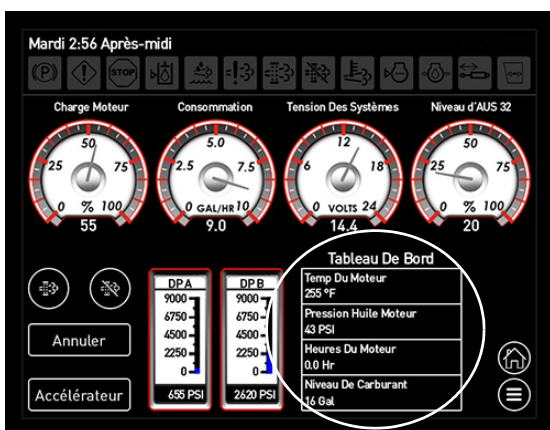
Diagnostic des systèmes (situés sur l'écran Diagnostique du moteur)
