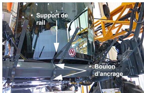
Ensemble du rail central du pare-broussailles - Vue typique
