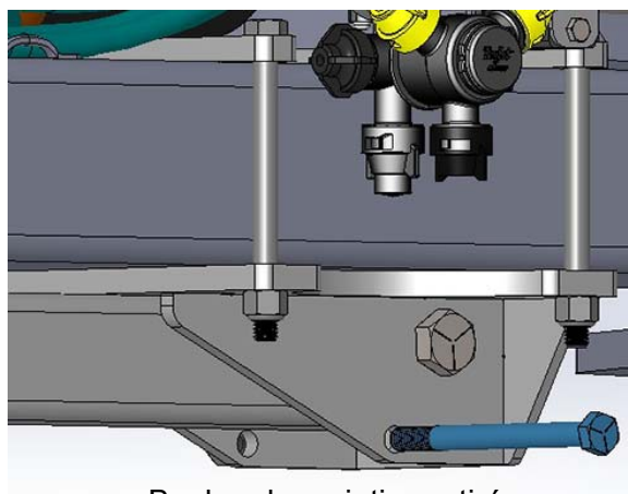
Boulon de maintien retiré - Vue typique
