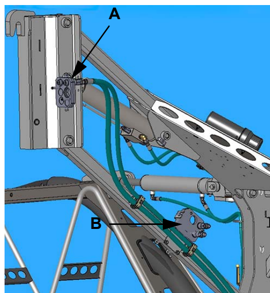
Dispositif de rangement de la poignée de raccordement rapide (situé sur le bras de relevage gauche de la rampe) - Vue typique
