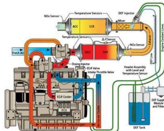
Système de postcombustion du moteur
