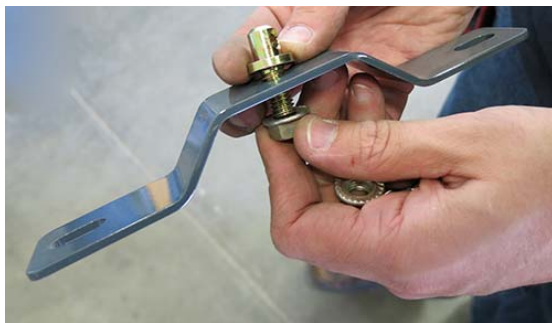
Matériel du support de fixation - Vue typique
