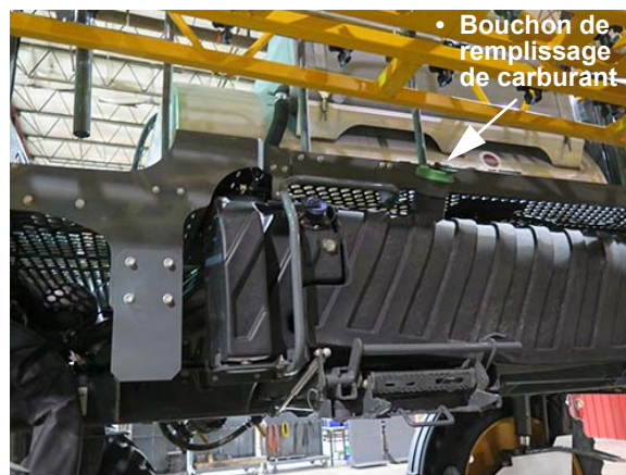
Remplissage de carburant (situé sur le haut du réservoir de carburant, du côté droit de la machine) - Vue typique
