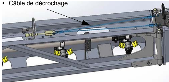
Décrochage de l'extension - Vue typique
