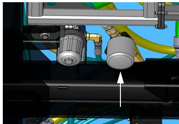
Filtre de retour au carter 2 (situé sur le côté gauche de la machine, à l'avant du châssis du moteur) - Vue typique
