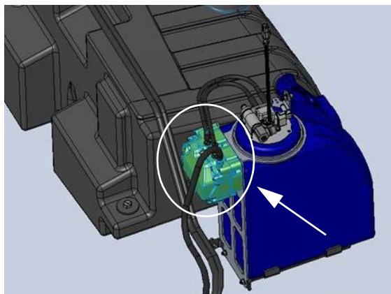
Module d'alimentation en AUS 32 (situé sur la partie arrière du réservoir d'AUS 32) - Vue typique
