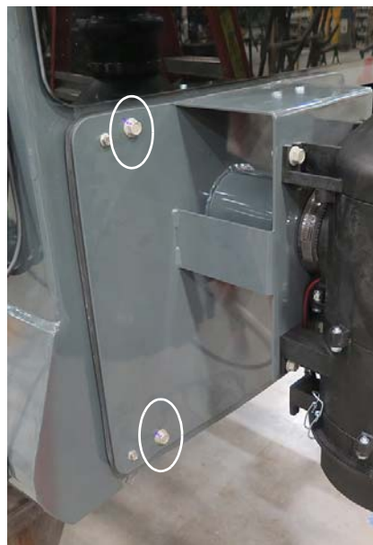
Boulons de fixation (4) (deux situés de chaque côté du panneau d'accès extérieur sur le côté droit de la cabine) - Vue typique
