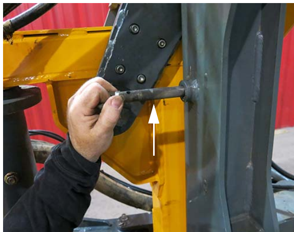
Boulon de fixation (situé sur la partie extérieure du châssis de la traverse) - Vue typique
