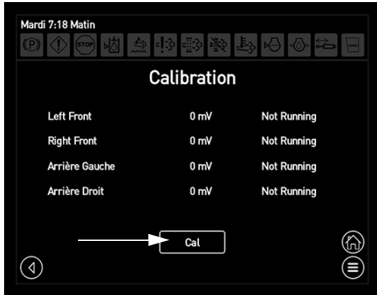
Touche Cal (située sur l'écran Calibrage)
