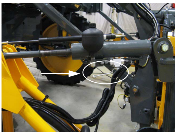
Vannes manuelles NORAC (2) (situées sur les vérins de mise de niveau gauche et droit) - Vue typique
