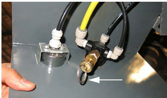
Anneau de traction de décharge de la pression (situé sur la partie arrière du régulateur de pression du mousser) - Vue typique
