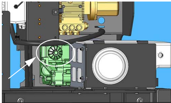
Filtre du module d'alimentation en AUS 32 (situé sous le module d'alimentation en AUS 32 - accès par le dessus de la machine) - Vue typique
