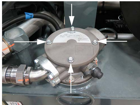
Boîtier du filtre de retour (situé sur le dessus du réservoir d'huile hydraulique) - Vue typique
