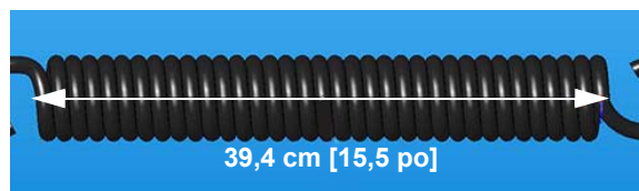
Décrochage à ressort - Vue typique
