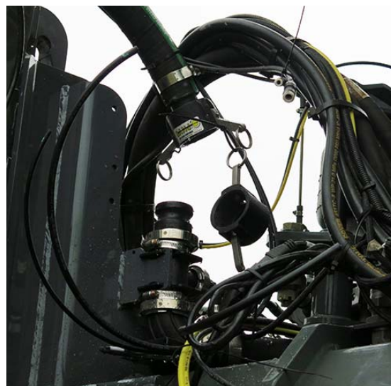
Branchement du système de solution - Standard (situé sur le côté avant droit de la machine) - Vue typique
