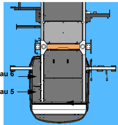
Installation du bouclier de bas de caisse arrière - Vue typique
