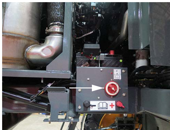
Sectionneur général de la batterie (situé à l'intérieur du compartiment moteur, du côté arrière droit de la machine - ouvrez le capot pour y accéder) - Vue typique
