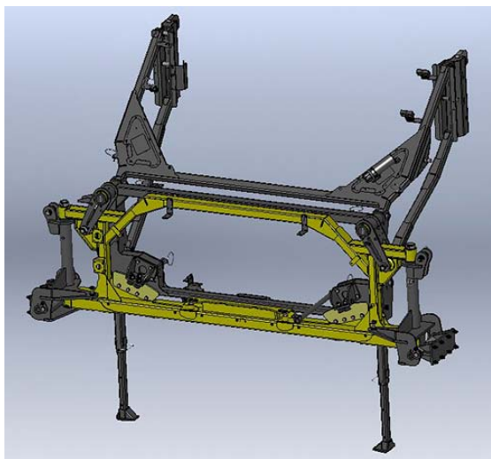
Chandelles de support de la rampe (rampe de 40 mètres) - Vue typique
