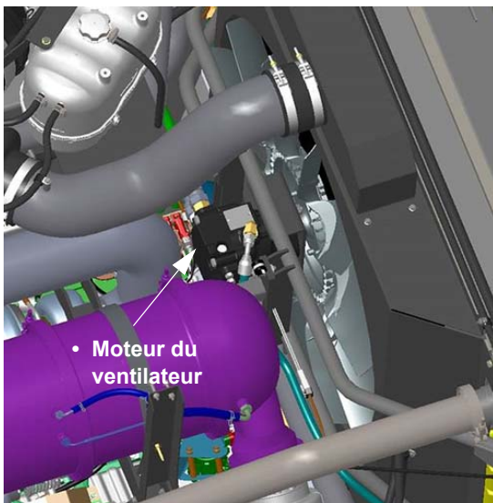
Ventilateur réversible (situé vers l'arrière de la machine) - ouvrez le capot pour y accéder) - Vue typique
