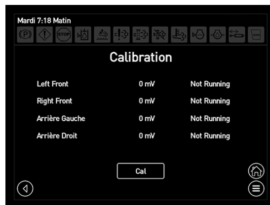
Touche Cal (située sur l'écran Calibrage)
