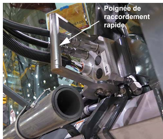
Ensemble multicoupleur hydraulique/électrique (situé sur le côté avant gauche de la machine) - Vue typique
