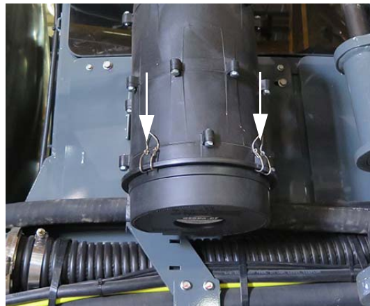
Loquets du filtre - Vue typique
