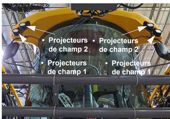
Projecteurs de champ (4) (situés à l'avant de la cabine) - Vue typique
