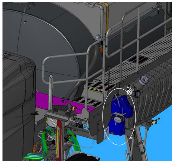
Réservoir d'AUS 32 (situé sur le côté droit de la machine, à proximité du réservoir de carburant) - Vue typique
