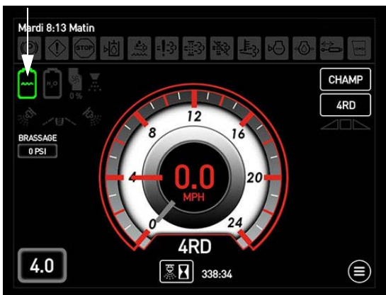
Voyant du réservoir principal (situé sur la page d'accueil de l'afficheur de la machine - mode Champ)
