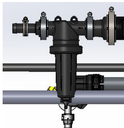
Crépines de sections (Situées tout au long des diverses sections de la rampe) - Vue typique
