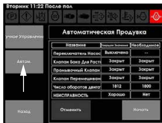
Экран продувки
