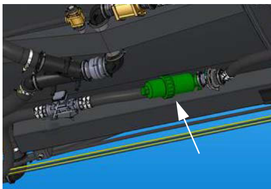
Сетчатый фильтр затворной линии (расположен в центре под правой стороной машины) - стандартный вид
