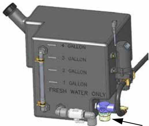
Сито ручмойника (расположенное возле нижней части бака ручмойника) - стандартный вид
