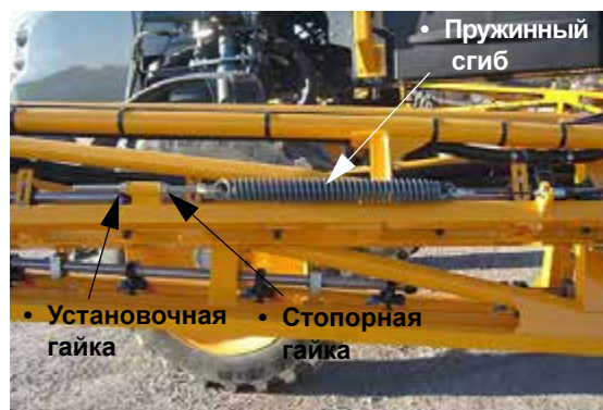
Регулировочные/Стопорные гайки пружинного сгиба (возле внешнего конца пружинного сгиба) - стандартный вид
