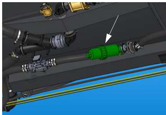
Сетчатый фильтр затворной линии (расположен снизу с правой стороны машины) - стандартный вид
