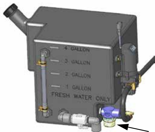
Сито ручмойника (расположено возле нижней части бака ручмойника) - стандартный вид
