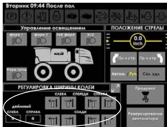
Кнопки/Индикаторы регулировки ширины колеи (находятся на Странице вспомогательных органов управления)
