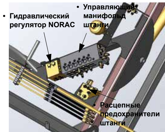
Управляющий manifold штанги и гидравлический регулятор NORAC – если поставлен (расположен на подъемном рычаге штанги в сборе) - стандартный вид
