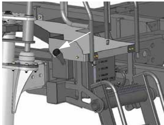
Заправочное отверстие рукомыльника (расположено под платформой рядом с лестницей) - стандартный вид
