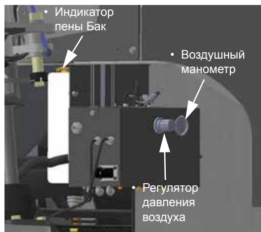
Блок управления индикатора пены (расположен под платформой на задней правой стороне машины) - стандартный вид
