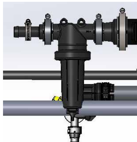
Сетчатый фильтр секции (расположен на каждой секции штанги) - стандартный вид
