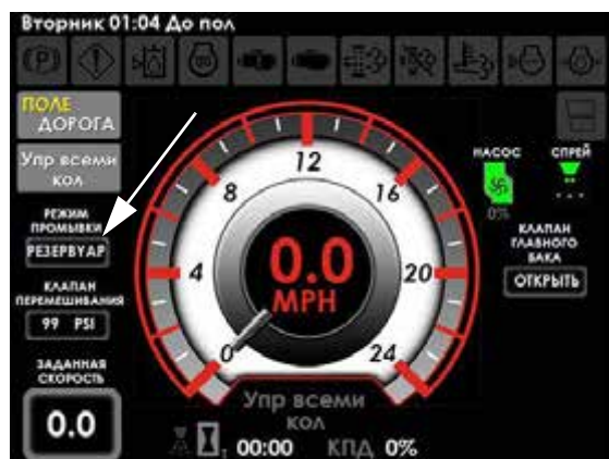
Индикатор режима промывки (расположен на Главной странице дисплея машины – в Полевом режиме)
