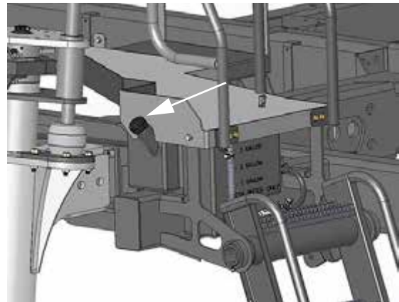
Заправочное отверстие рукомойника (расположенное возле лестницы) - стандартный вид
