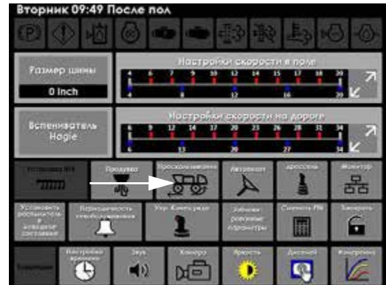
Кнопка пробуксовки (расположена на Странице настроек)
