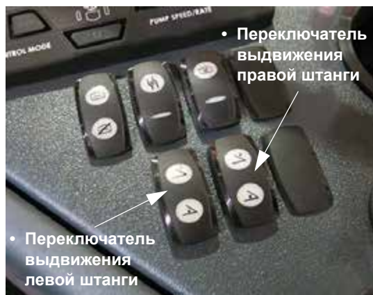
Переключатели выдвижения левой и правой штанг (расположен на боковой панели) - стандартный вид
