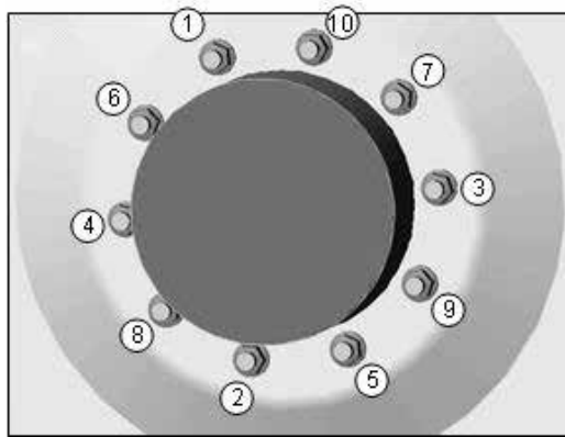
Очередность затяжки
