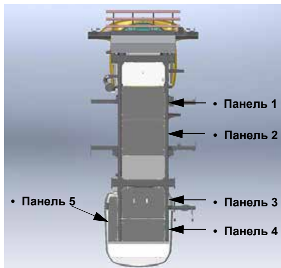
Установка утолщающей накладки – стандартный вид * Показан вид снизу машины
