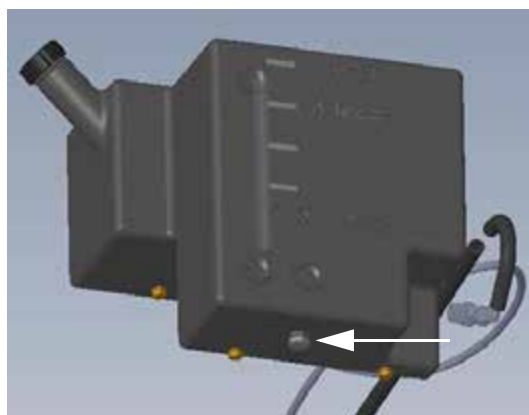
Спускная пробка (расположена под рукомоинным баком) - стандартный вид
