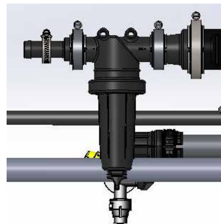
Сетчатые фильтры секции (расположены на каждой секции штанги) - стандартный вид
