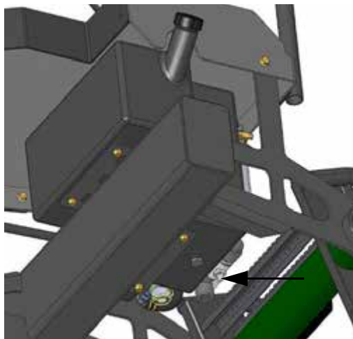
Вентиль рукомыльника (расположен возле нижней части бака рукомыльника) - стандартный вид
