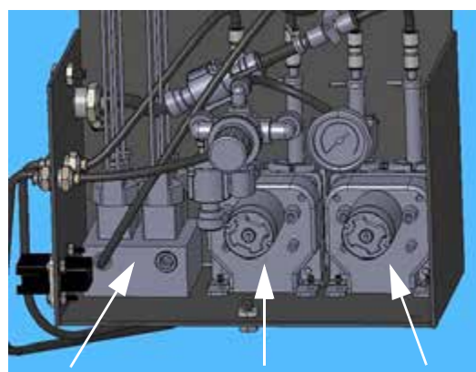
• Коллектор • Насос для концентрата • Водяной насос
