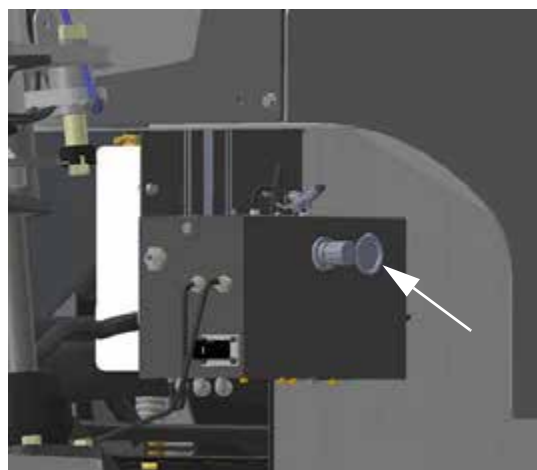
Воздушный манометр (расположен на Блоке управления индикатора пены) - стандартный вид
