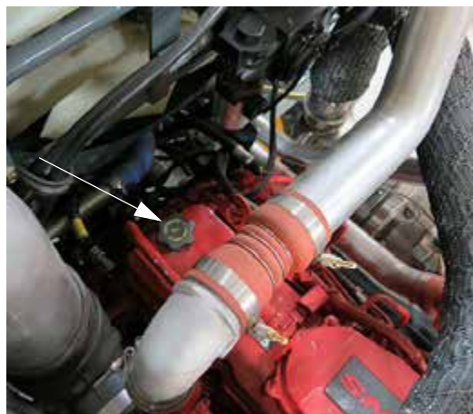
Заливка моторного масла (расположена сверху двигателя) - стандартный вид
