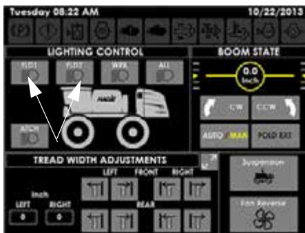
Кнопки полевого освещения (находятся на странице вспомогательных органов управления)
