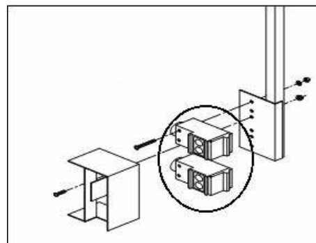
LS-фотодатчики (верхний/нижний) - стандартный вид
