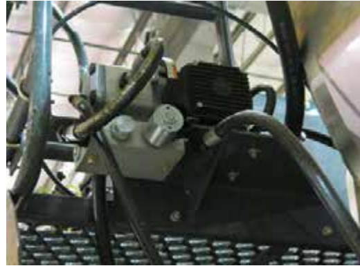
Nagynyomású tisztító szivattyú (a gép jobb oldalán hátul) – Tipikus nézet
