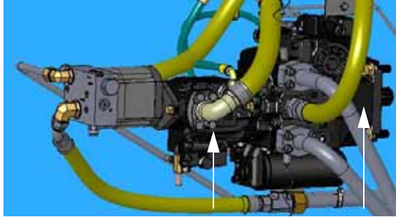
Bombas hidrostáticas -Vista típica
