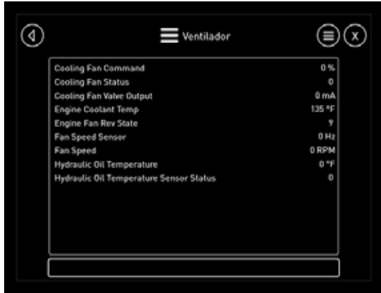
Pantalla Grupo de medidas
