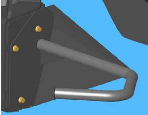
Conjunto del divisor de cultivos -Vista típica
