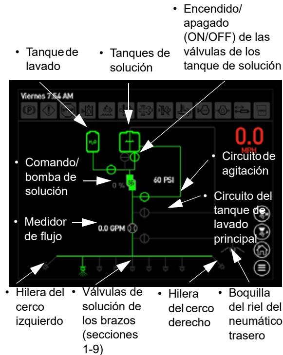
Pantalla Esquema del Sistema de soluciones
