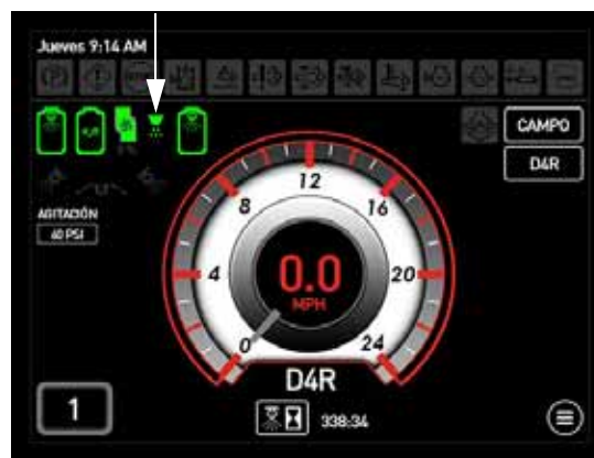
Indicador de aspersión principal (ubicado en la parte superior derecha de la página principal de la pantalla de la máquina - modo de campo)
