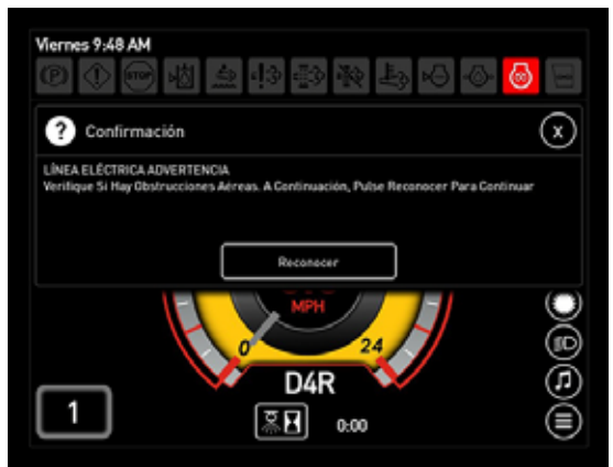
Mensaje de advertencia de línea de alta tensión (en la pantalla de la máquina)
