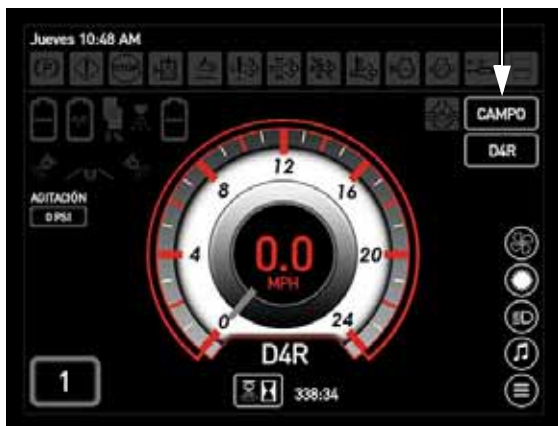
Botón de campo/carretera (página principal - modo de campo)
