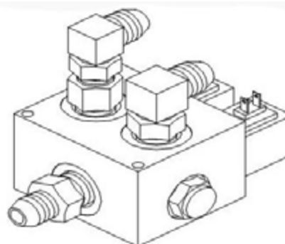
Distributeur de traction - Vue typique
