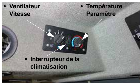
Commandes de climatisation (situées au plafond de la cabine) - Vue typique
