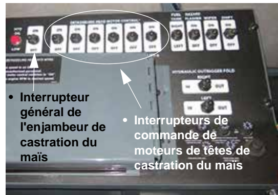
Interrupteur général de l'enjambeur de castration du maïs et boutons de gestion des moteurs des têtes de castration du maïs (situés sur le montant droit) - Vue typique
