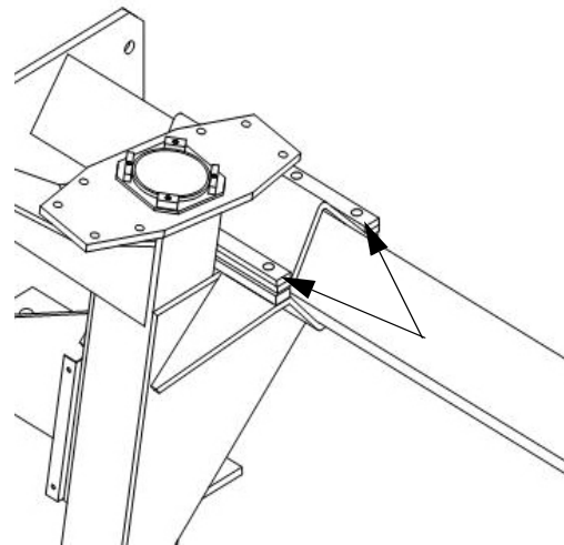
Boulons de fixation des jambes (six sur chaque jambe) - Vue typique
