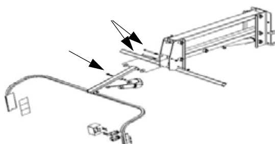
Boulons de pivot du LS pour contrôle de la profondeur - Vue typique
