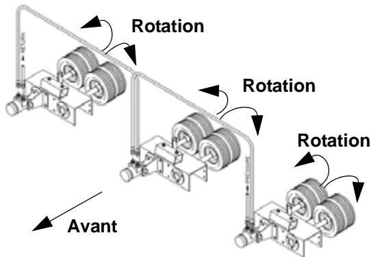
Assemblage hydraulique des arracheuses de fleurs (modèle à trois têtes) - Vue typique
