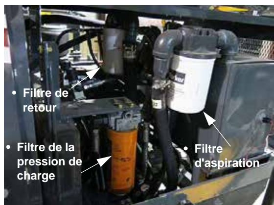
Filtres d'aspiration, de pression de charge, et de retour (situé près du côté arrière gauche de la machine - ouvrir le capot du moteur pour y accéder) - Vue typique
