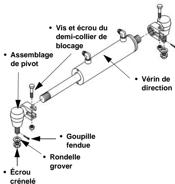
Assemblage du vérin de direction - Vue typique
