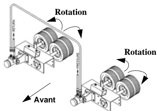
Assemblage hydraulique des arracheuses de fleurs (modèle à deux têtes) - Vue typique
