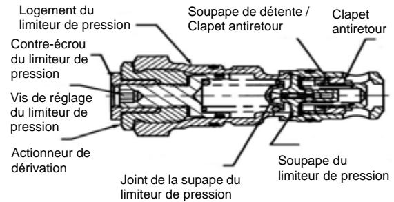
Coupe transversale d'une soupape multifonctions
