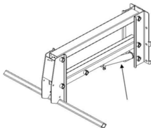
Vérins de relevage (situés sur chaque bras de module) - Vue typique
