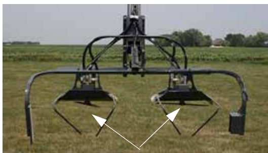
Têtes de coupe - Vue typique
