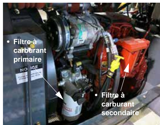
Filtres à carburant primaire et secondaire (situés sur le côté gauche du moteur - ouvrir le capot du moteur pour y accéder) - Vue typique
