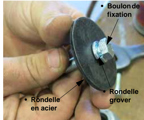
Assemblage boulon de fixation et rondelle d'une lame de coupe - Vue typique
