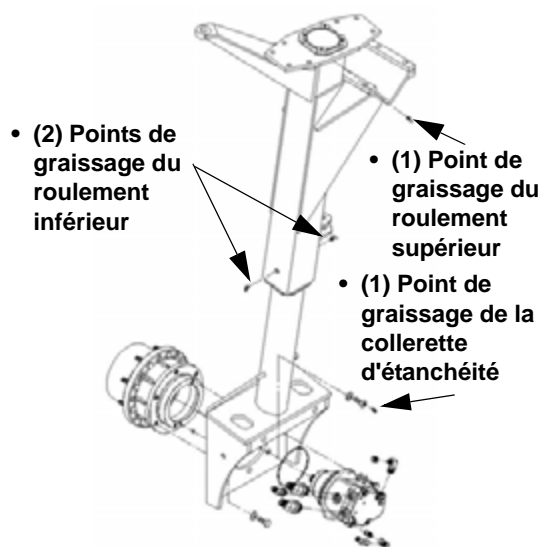
Points de graissage du roulement de jambe et de la collerette d'étanchéité du Torque Hub - Vue typique
