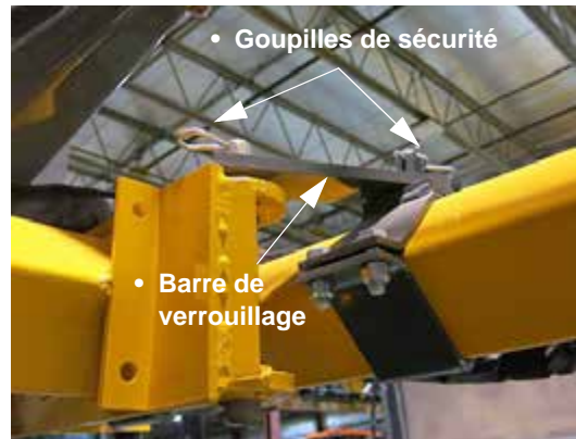
Assemblage goupille de sécurité-barre de verrouillage (situé entre la rampe et la barre porte-outils centrale) - Vue typique
