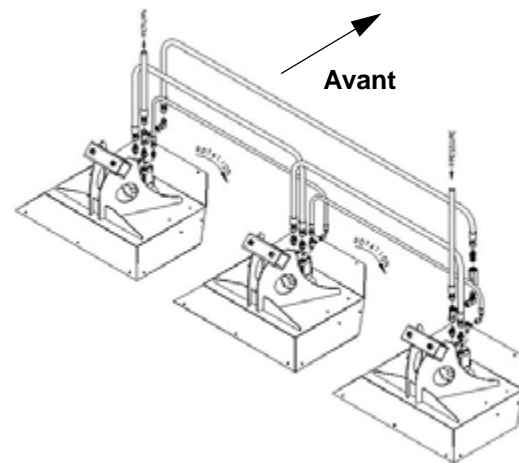
Rotation de la lame - À gauche de l'opérateur (modèle à trois têtes) - Vue typique
