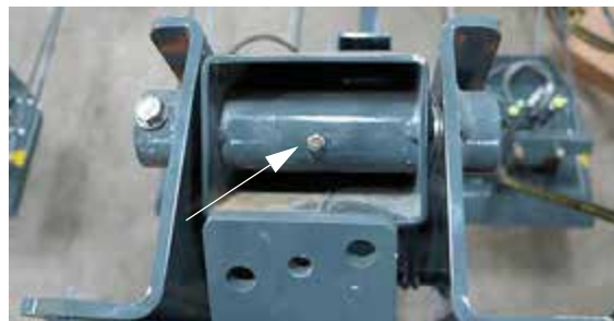
Assemblage d'un bras de relevage - Section supérieure - Vue typique
