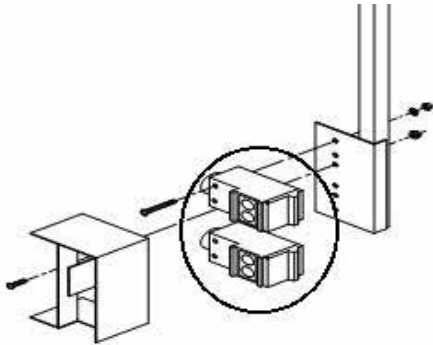
Photocellules du système LS (haut / bas) - Vue typique
