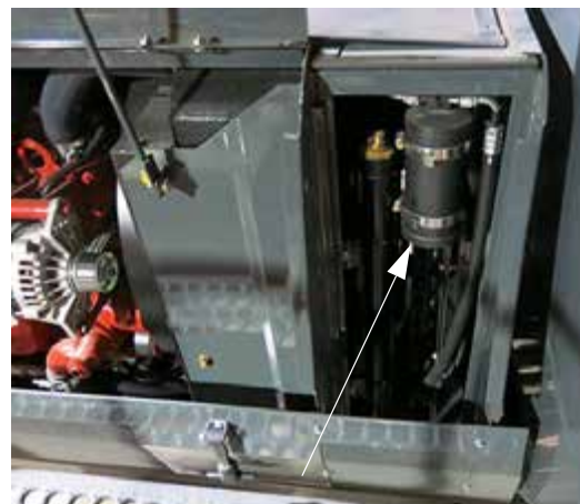
Récepteur-déshydrateur du circuit de climatisation (situé derrière la cabine, près du radiateur - déposer les écrans du radiateur pour y accéder) - Vue typique
