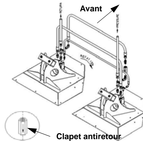
Rotation de la lame - À gauche de l'opérateur (modèle à deux têtes) - Vue typique
